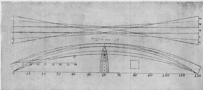
1. Схема расположения ферм деревянного арочного моста (фасад и план), с проекцией арок, разбитой на 120 частей. См. Описание, № 11.
