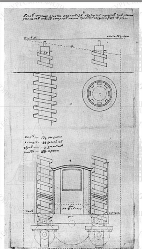
180. «Подъемные кресла» (общий вид спереди, боковой вид части винта и план гайки).
