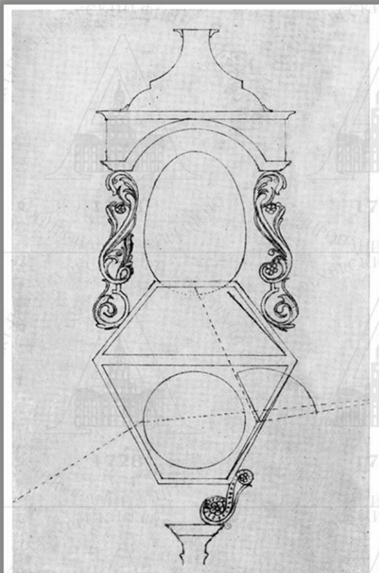
76. Подставка к часам «яичной фигуры» с системой зеркал для наблюдения за показаниями стрелок без переворачивания часов (боковой вид). См. Описание, № 264.
