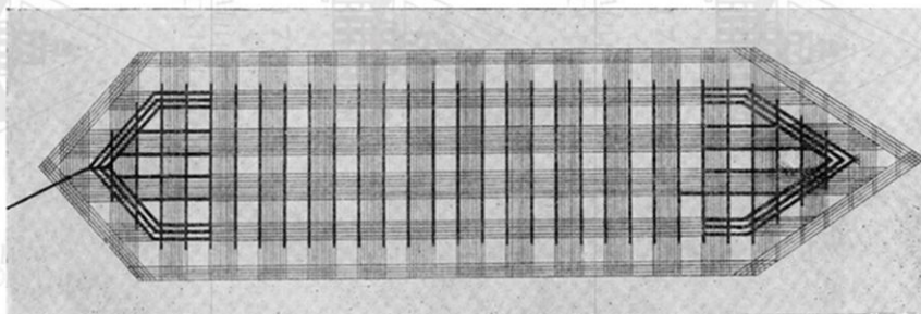
21. Очертание промежуточной опоры (план). см. Описание, № 65.
