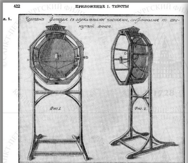
Фонарь с зеркальным отражателем.
