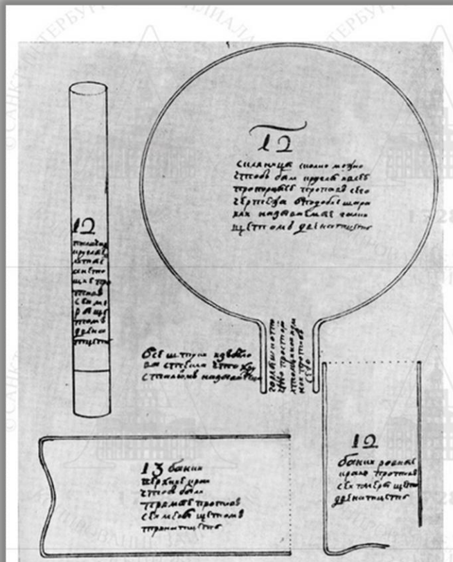
147. Рабочие чертежи стеклянных деталей шаровой переносной электрической машины. См. Описание, № 509.
