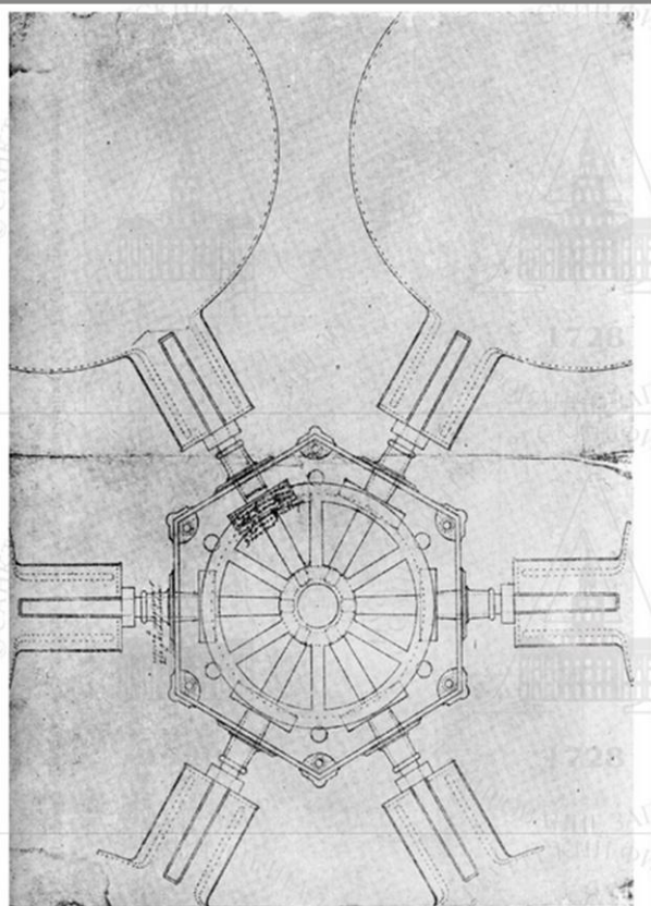
143. Электрическая машина с шестью шарами (разрез). См. Описание, № 505.
