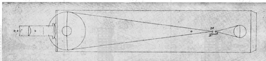
110. Зеркальный телескоп со схемой расположения зеркал и линз окуляра. См. Описание, № 356.
