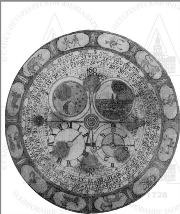
90. Рисунок циферблата карманных планетных часов с изображением знаков зодиака. См. Описание, № 312.
